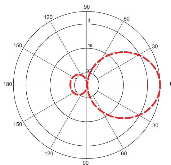
Antenna vertikális karakterisztika (E-plane)
